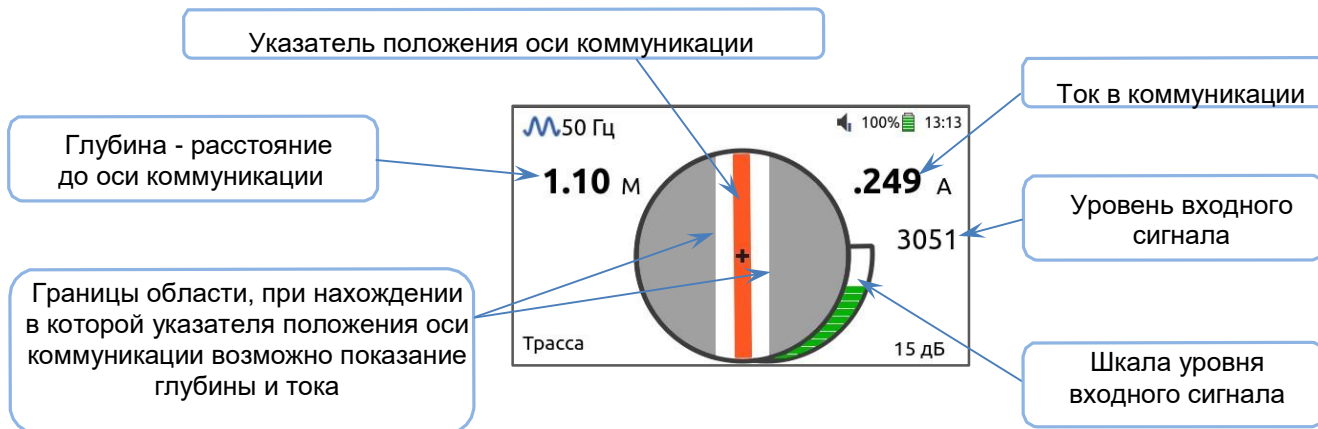
Рисунок 3.3. Экран приемника в режиме «Трасса».
