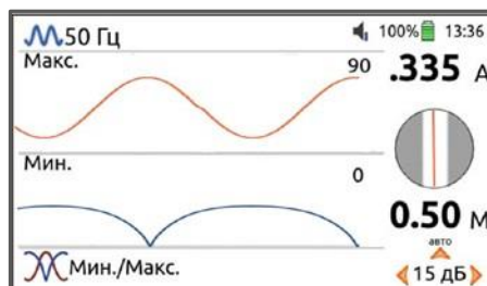
Рисунок 3.13. Режим индикации «Мин./Макс.».
