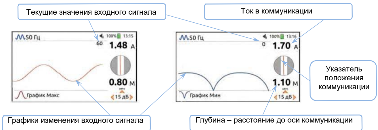
Рисунок 3.12. Режимы «График Макс» и «График Мин».
