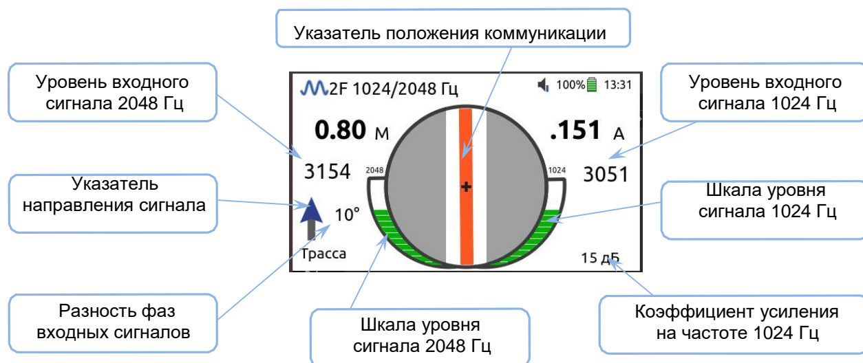
Рисунок 3.14. Режим «Трасса» при двухчастотном режиме.
