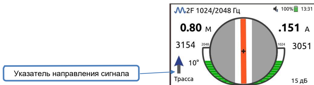
Рисунок 3.17. Указатель направления сигнала в режиме «2F 1024/2048».
