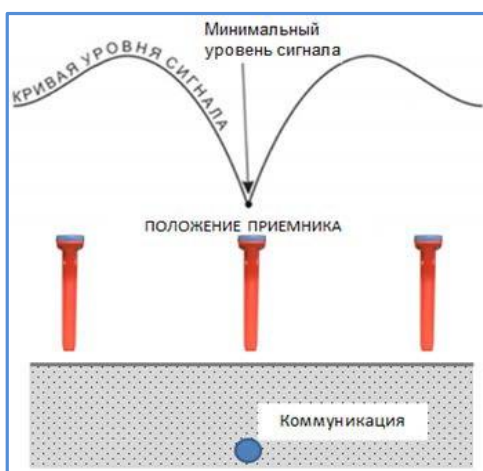
Рисунок 3.9. Метод «минимума».
