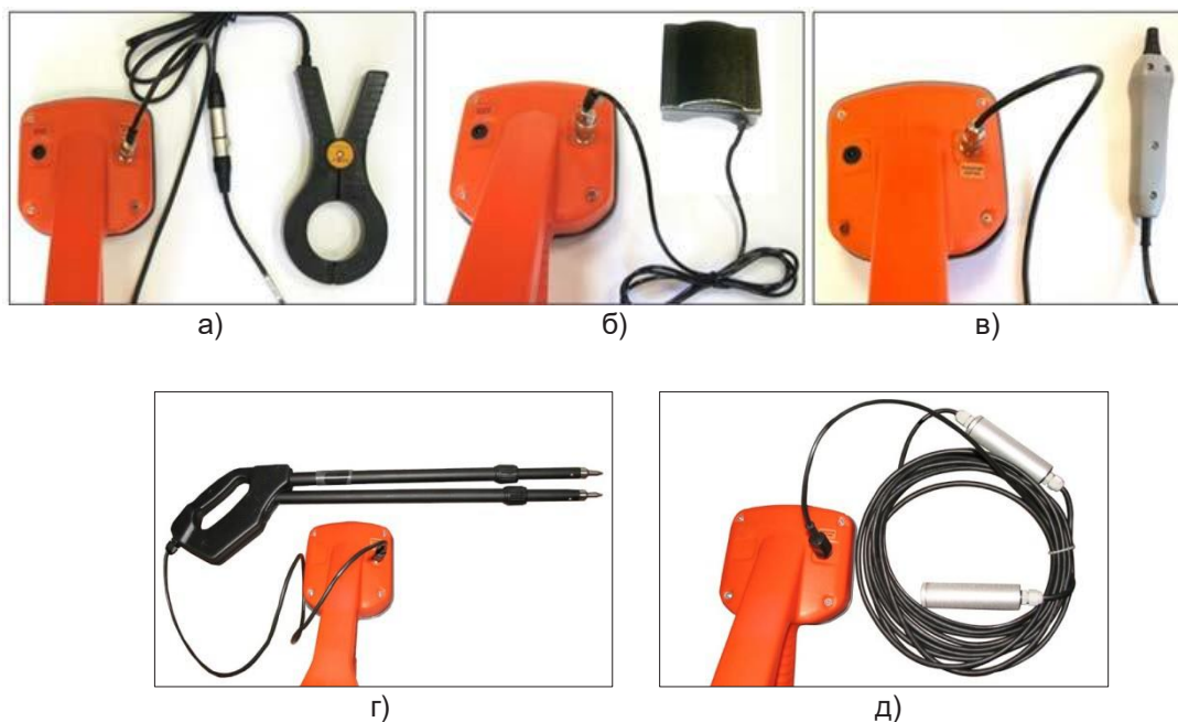
Рисунок 6.1. Подключение внешних датчиков.
