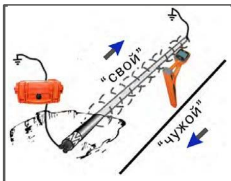
Рисунок 3.16. «Свой» и «чужой» сигналы в коммуникациях.
