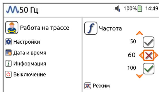
Рисунок 4.7. Выбор рабочих частот в разделе меню «Частота».
