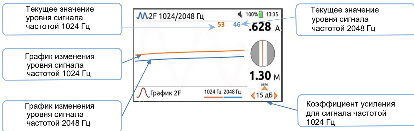
Рисунок 3.15. Режим индикации «График 2F».
