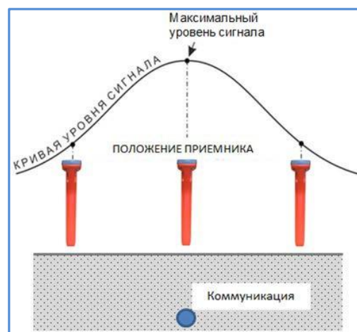
Рисунок 3.10. Метод «максимума».
