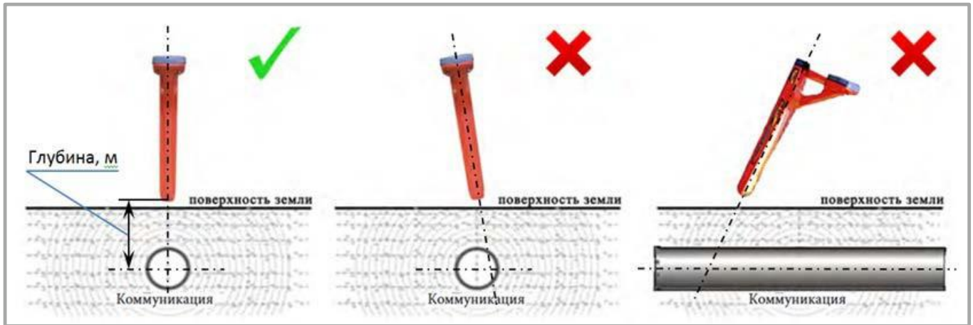
Рисунок 3.5. Правильное положение приемника при замере глубины.
