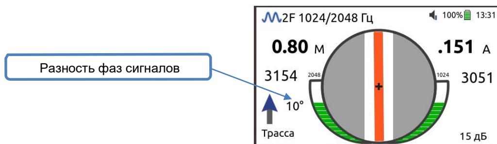
Рисунок 3.18. Параметр «Разность фаз» в двухчастотном режиме.
