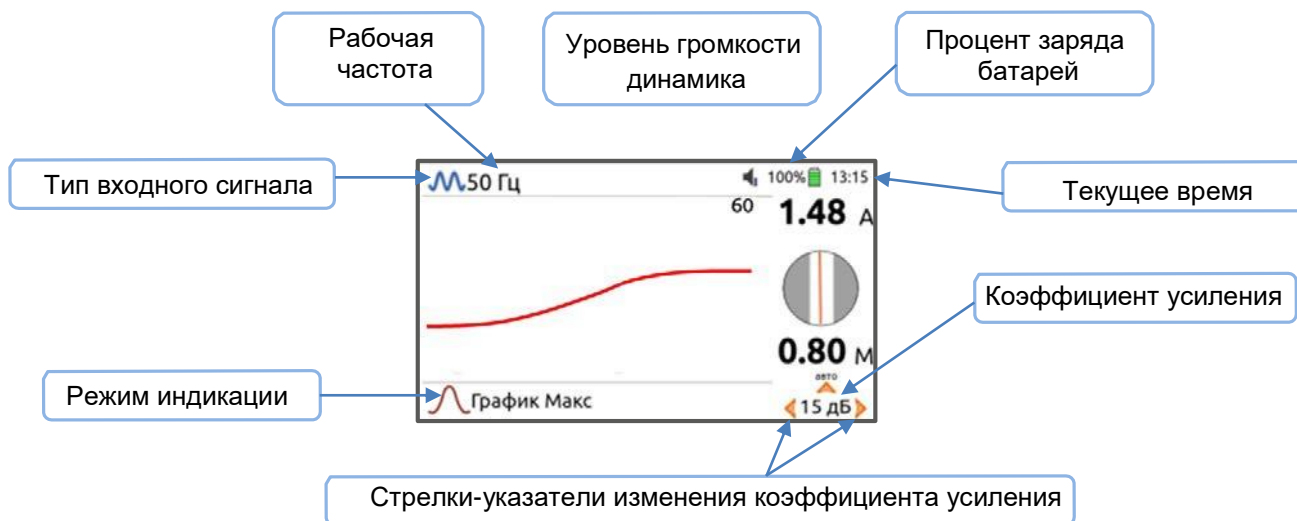
Рисунок 3.2. Вид экрана в режиме «График Макс».
