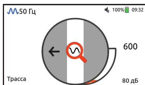
Рисунок 3.8. Экран приемника в режиме «Трасса» при слабом сигнале. Уточнить положение коммуникации в этом случае можно в режимах «Пик», «Ноль» или «Мин./Макс».
